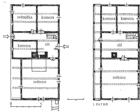
Obr. č.7 půdorys čp.75 v Novoměstské ulici repro: Mencl, V., doc.Dr.Ing.arch.: Lidová architektura v Československu, Academia, Praha, 1980, str.237
